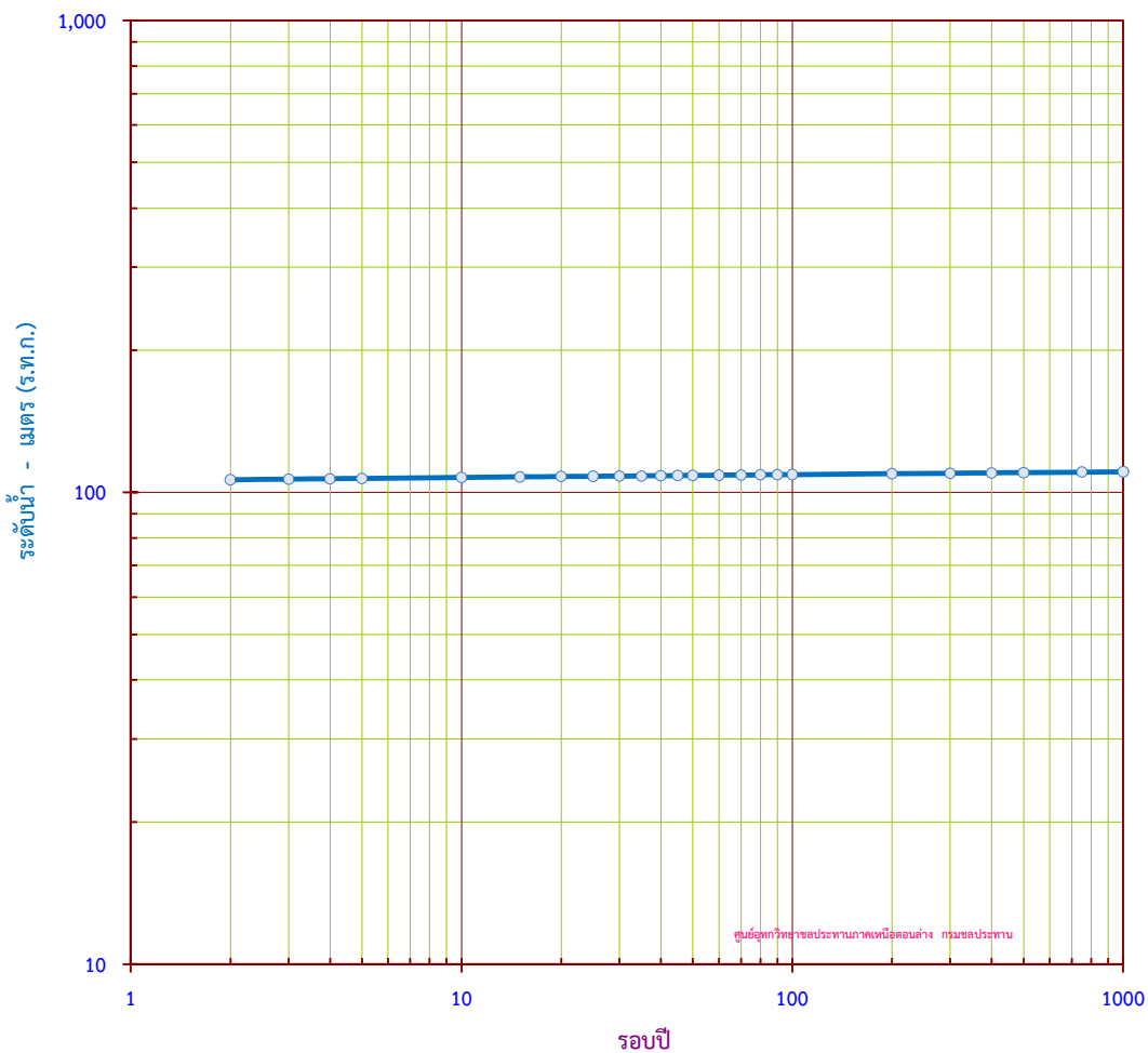
กราฟแสดง ระดับน้ำสูงสุดรายปี ขนาดรอบปีต่างๆ สถานี P.2A อ.เมือง จ.ตาก
